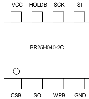
Figure 6. 端子配置図
