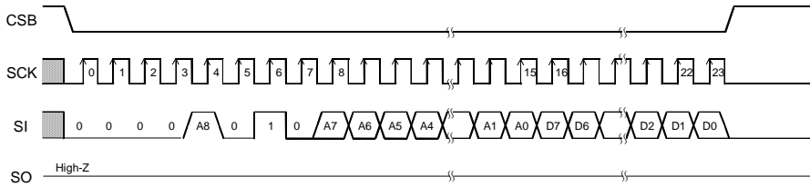
Figure 38. 書き込み命令
